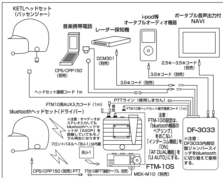
<接続図5>Bluetoothヘッドセット（ドライバー） +有線ヘッドセット（パッセンジャー）タンデム接続
