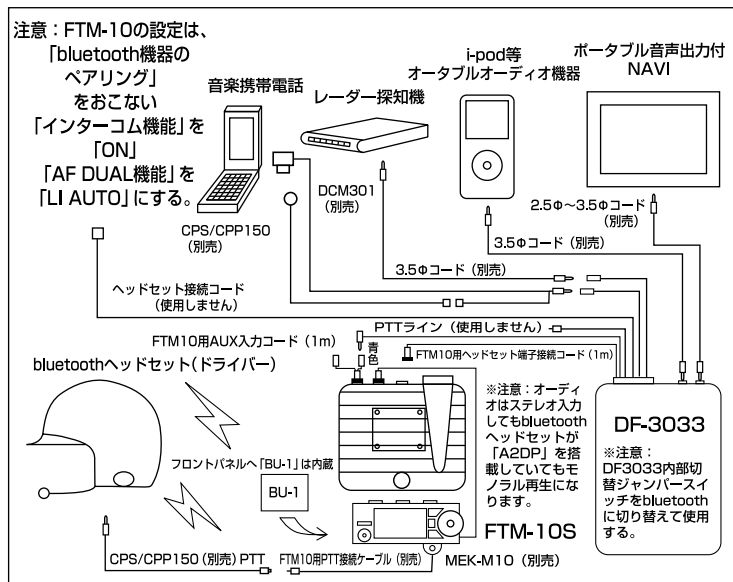
<接続図4>Bluetoothヘッドセット接続
