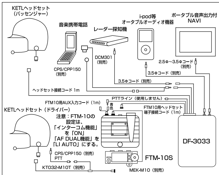
<接続図3>有線タンデム接続
