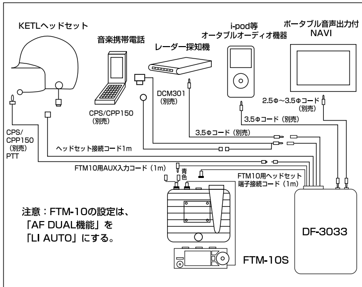
<接続図1>有線シングル接続
