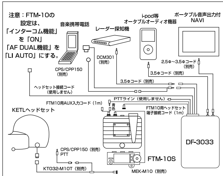
<接続図2>有線シングル接続（フロント接続）
